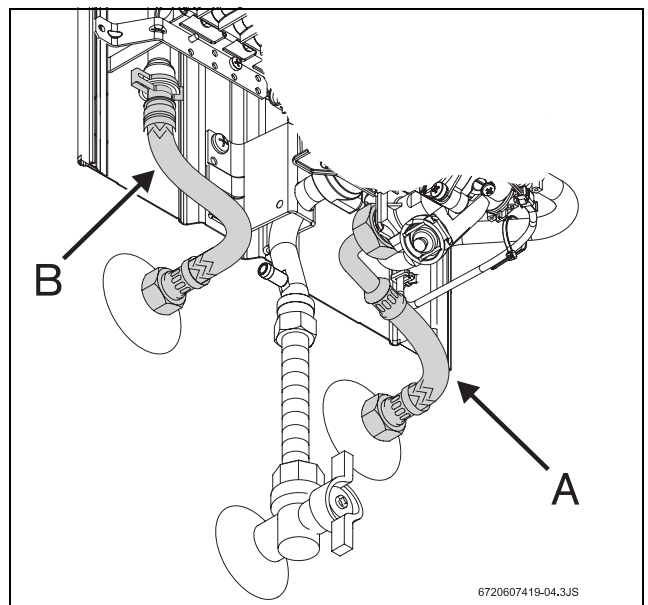
Рис 4 Подключение водопровода
